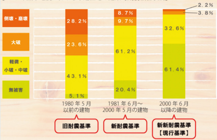
【2016年熊本地震における木造住宅の建築時期別被害状況】
