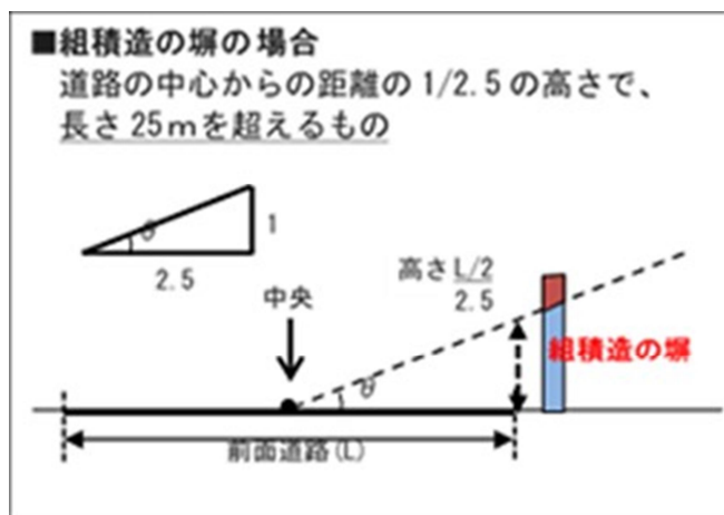
図 2-2 通行障害建築物となる組積造の塀
